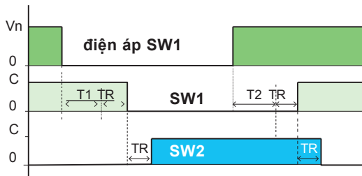
ATS nguồn Lưới: Chế độ tự động (vận hành song song sau khi tự động chuyển nguồn)
