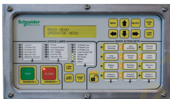
Giao diện vận hành flexVUE
