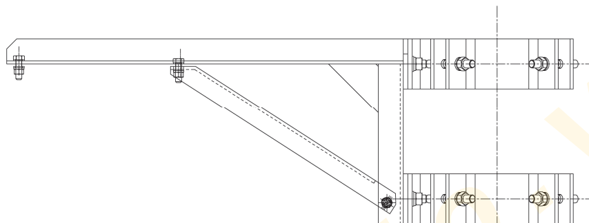
Bộ giá đỡ gá lắp 27 kV/38 kV (Cùng loại giá đỡ cho kiểu gá lắp lệch bên và ở giữa)
