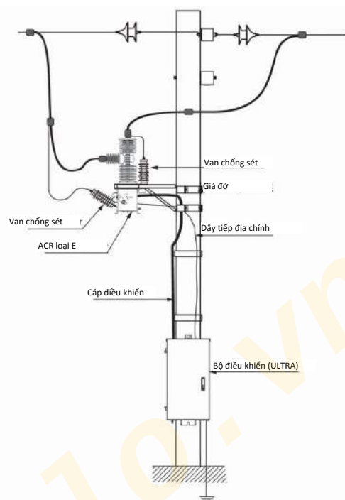
Ví dụ lắp đặt kiểu ở giữa cho loại 38 kV
